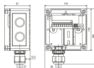
Maßbild DCU EMOB 2 16
