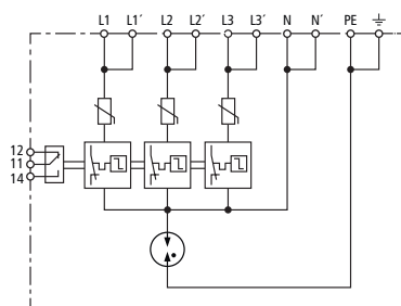
Prinzipschaltbild DCU EMOB 2 16
