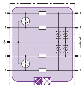
Prinzipschaltbild BXT ML4 BE 36
