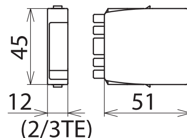
Maßbild BXT ML4 BE 36
