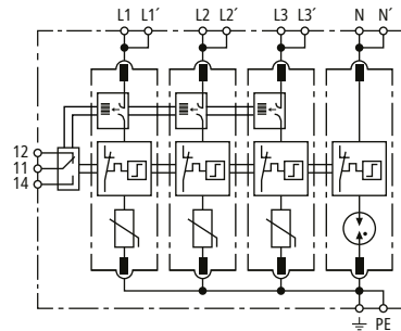
Prinzipschaltbild DG MP TNS ACI 275 FM
