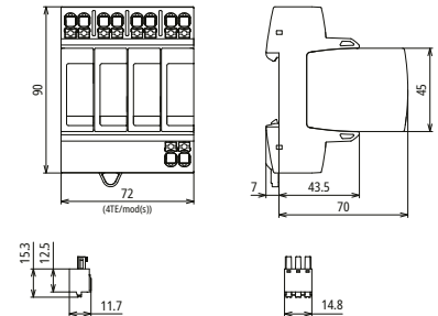
Maßbild DG MP TNS ACI 275 FM
