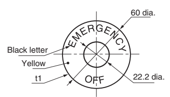
A22Z-3466-2 (60 dia.)
