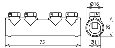
Maßbild VM 7.10 SKM6X12 ZG
