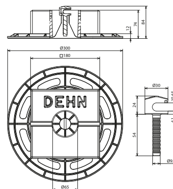
Maßbild DLH 8.10 KS BES180 GP300 K
