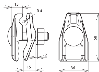
Maßbild AK 7.10 FRM10X45 KBF0.4 12 TGTZN
