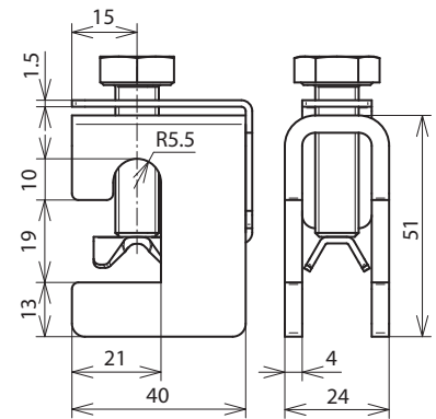
Maßbild AK 6.10 DS KBF5 18 STTZN
