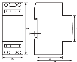
Maßzeichnung Gruppenansicht
