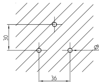
Bohrbild
