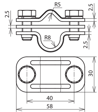
Maßbild UTK 200 8.10 16 ZP V2A
