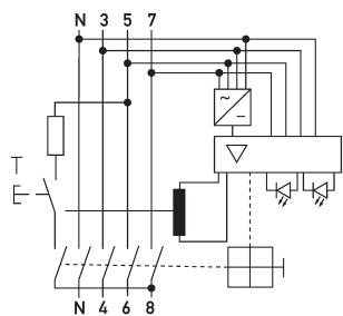
Schaltungsbeispiel Fehlerstromschutzschalter DFS 6 063-4/0,03-A NU
