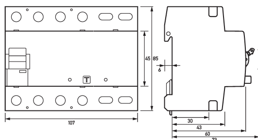
Maßzeichnung Fehlerstromschutzschalter DFS 6 063-4/0,03-A NU
