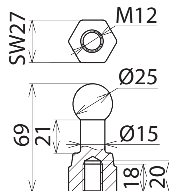
Maßbild KFP 25 M12
