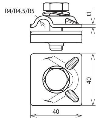
Maßbild MVK 8.10 SKM10X30 FSC AL
