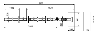
Maßbild IS 25 ZK RK 3160
