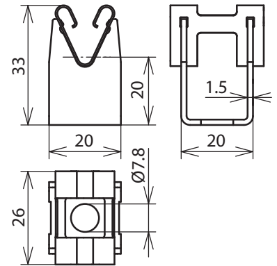
Maßbild LH DG 8 H20 B7.8 V2A
