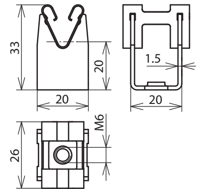
Maßbild
