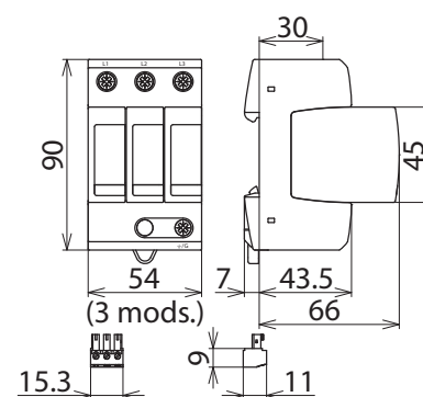
Maßbild DG MU 3PD 480 3W+G R
