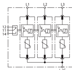
Prinzipschaltbild DG MU 3PD 480 3W+G R
