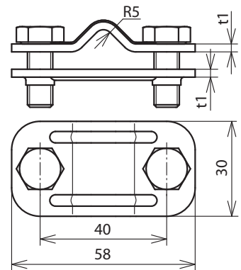
Maßbild UTK 8.10 FL30 V2A
