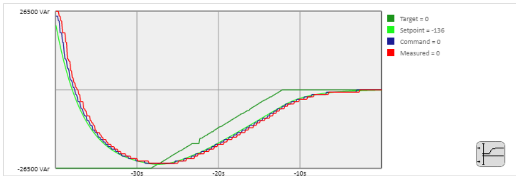
Abb.: Fließgrafiken (Auszugsweise) - Phasenverschiebung und Blindleistung mit Beispiel-Werten
