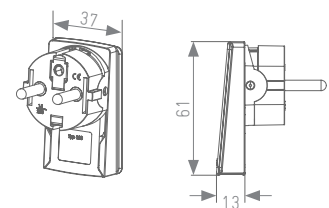
EVoline® PlugMini
