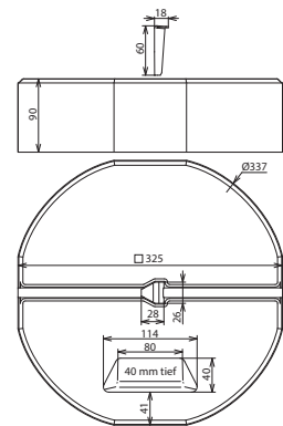
Maßbild BES 17KG KT16 D337 SET
