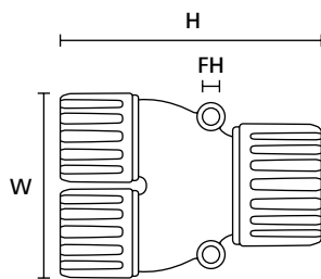
HelaGuard Verschraubung, Y-Verbinder
