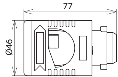
Maßbild CUI HEAD 20
