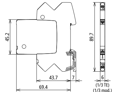
Maßbild BCO ML2 B 180
