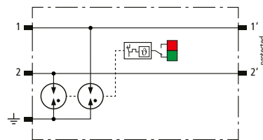
Prinzipschaltbild BCO ML2 B 180
