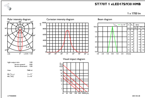
IFAS1_ST770T1xLED17S930HMB
