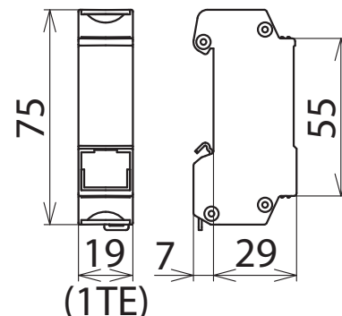
Maßbild DPA M CLD RJ45B 48
