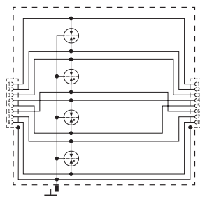
Prinzipschaltbild DPA M CLD RJ45B 48
