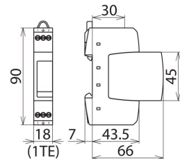
Maßbild DR M 2P 75
