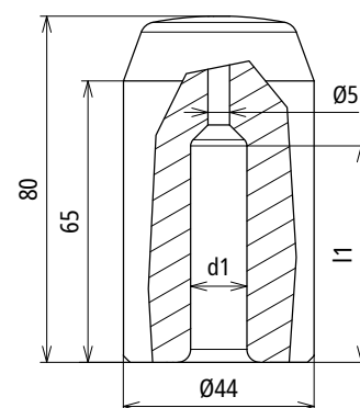
Maßbild SKO TE 25 STBLANK
