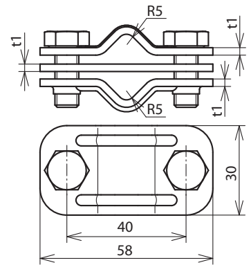
Maßbild UTK 8.10 8.10 ZP CU
