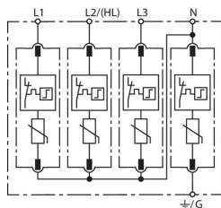
Prinzip Schaltbild DG MU 3PH 240 4W+G
