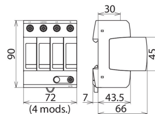
Maßbild DG MU 3PH 240 4W+G
