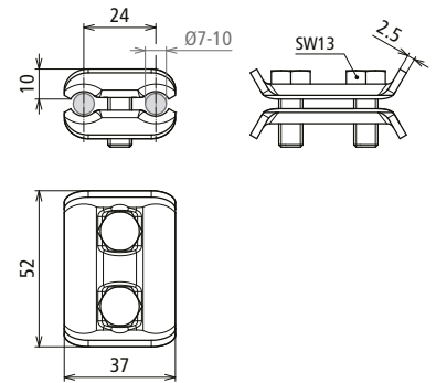
Maßbild PV 7.10 SKM8X20 STTZN
