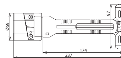
Maßbild HVI STRIP 27
