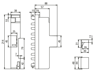
Maßbild DSH ZP 2 TNC 255
