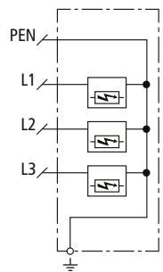
Prinzipschaltbild DSH ZP 2 TNC 255
