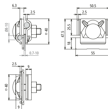
Maßbild FK MV 8.10 KBF0.7 10 V2A
