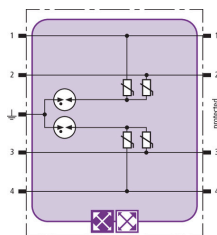
Prinzipialschaltbild BXT ML4 MY 110
