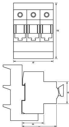
Maßzeichnung Gruppenansicht
