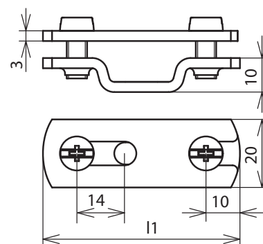
Maßbild FBH ZS 30 B6.5X16 STTZN
