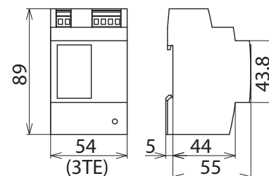
Maßbild PSU DC24 30W
