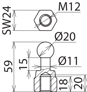
Maßbild KFP 20 M12
