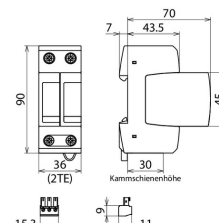
Maßbild DG M TT 2P ACI 275 FM
