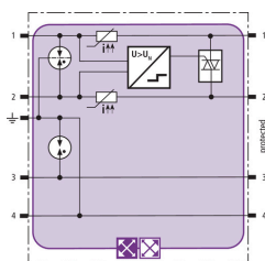
Principalschaltbild BXTU ML2 BD S 0-180
