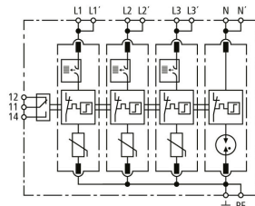
Prinzipialschaltbild DG MP TNS ACI 275 FM
