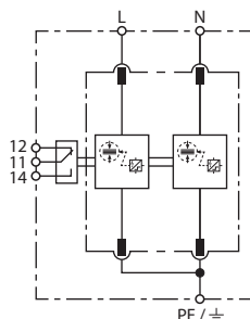
Prinzipialschaltbild DV M2 TN 255 FM
