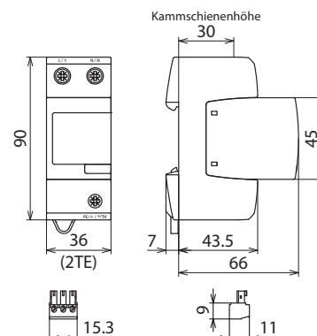
Maßbild DV M2 TN 255 FM
