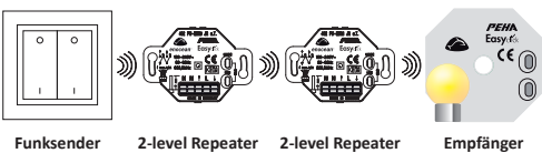
Funksender 2-level Repeater 2-level Repeater Empfänger
