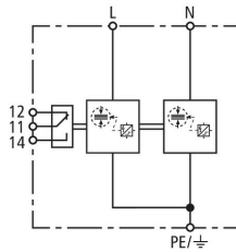
Prinzip Schaltbild DSH TN 255 FM
