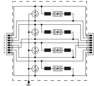
Prinzipschaltbild
