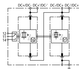
Prinzipschaltbild DSE M 2P 60 FM
