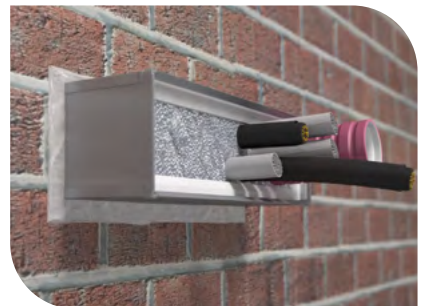
Wandeinbau
