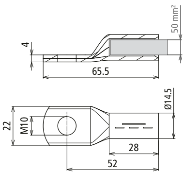
Maßbild PKS 50 10 CUGALNISN
